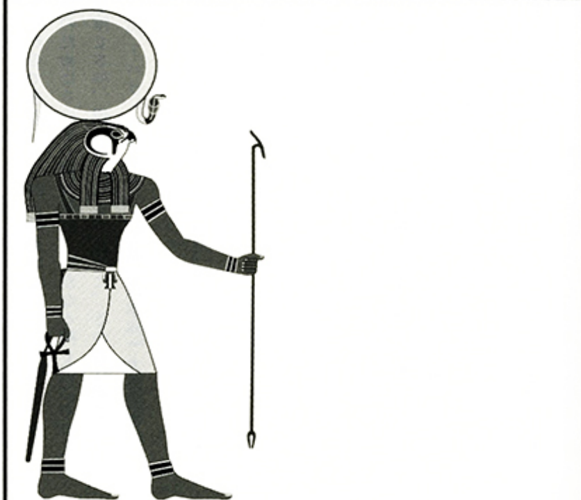
図21 ラメセス2世第神殿に掘られた太陽神ラー（ラー・ホルアクティ）とラー神の模式図
